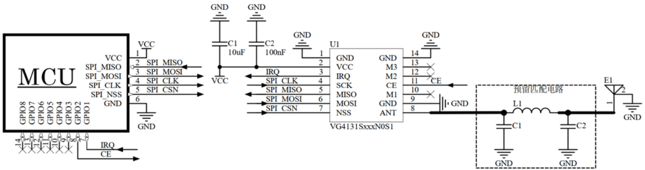
图 5-1 编程开发硬件连接
