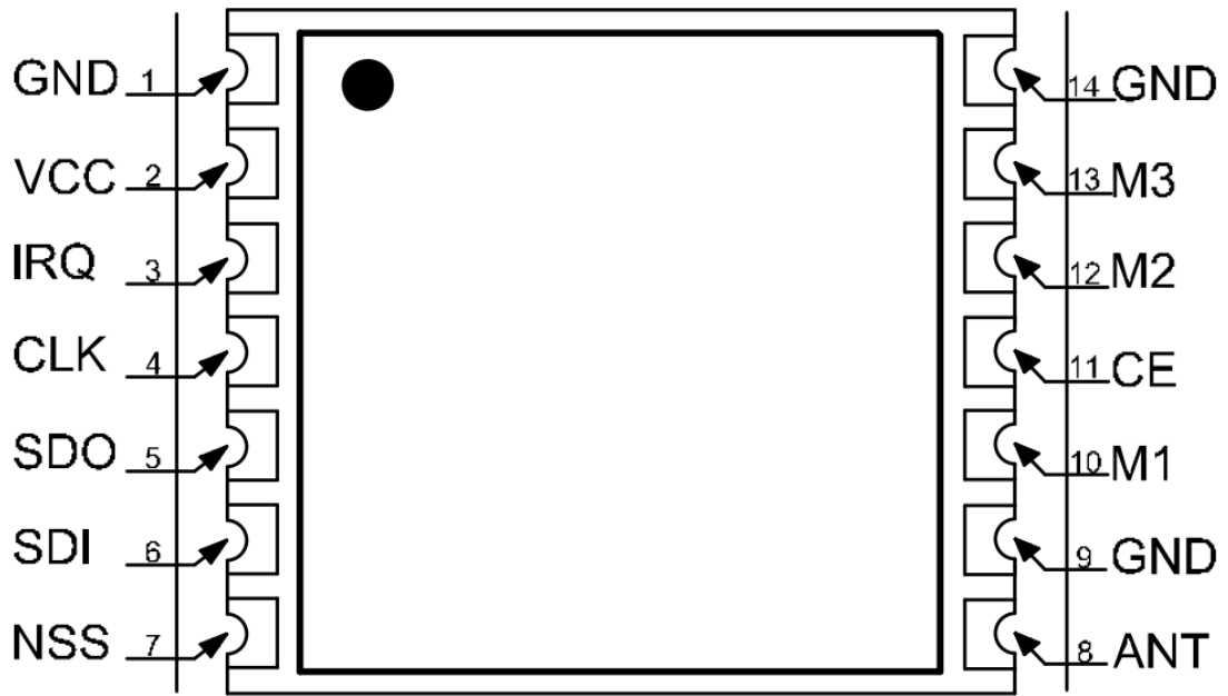
图 1-1 俯视图
