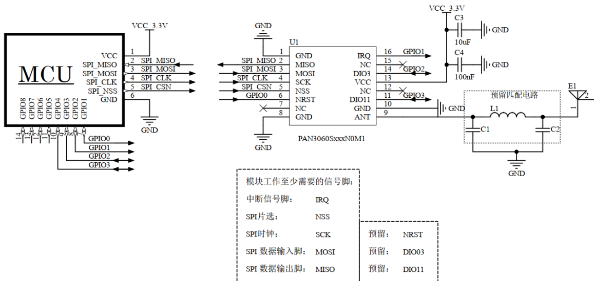
图 5-1 编程开发硬件连接
