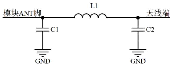
5-2 \pi 型匹配电路
