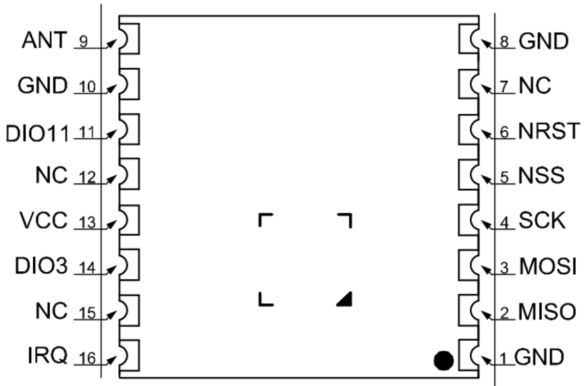
图 3-1 俯视图
