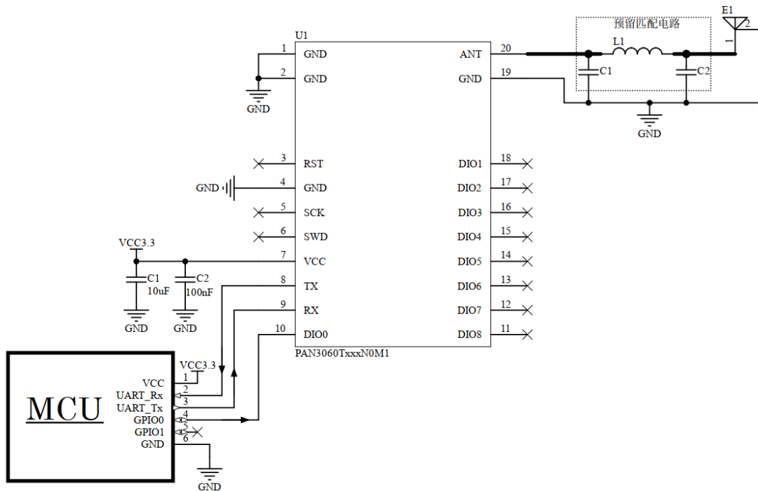
图 5-1 编程开发硬件连接
