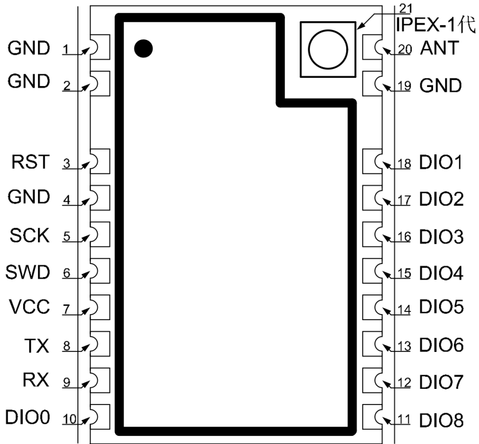
图 3-1 俯视图
