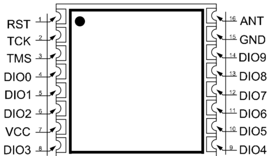
图 1-1 俯视图
