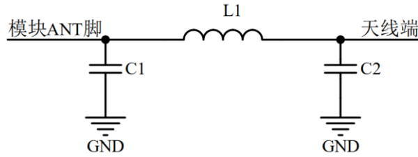
5-2 \pi 型匹配电路
