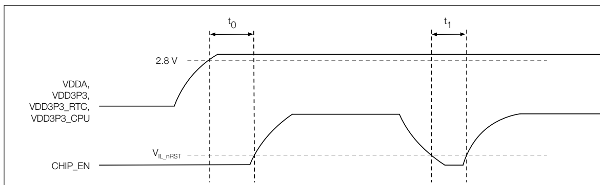
图 5: ESP32-C3 系列芯片上电、复位时序图
