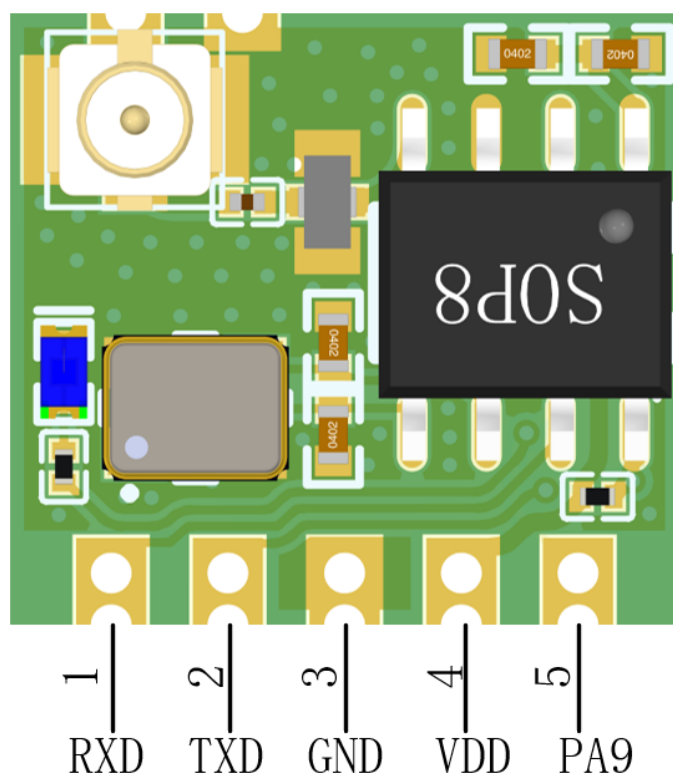
图 3-2：模组引脚
